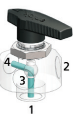
端口1,4连通
