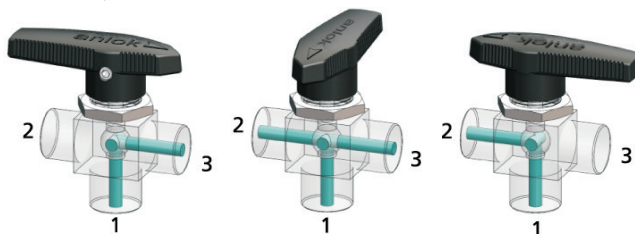
端口1,3连通
