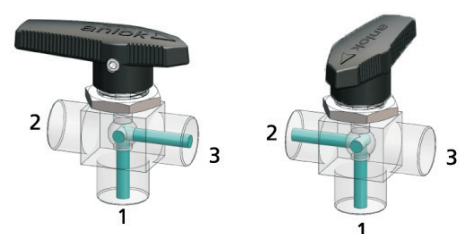
端口1,3连通
