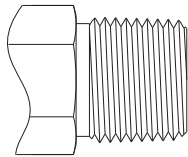
牙型角55° 以英寸为单位测量螺距 牙底和牙顶的截面是圆弧的 锥度1：16
