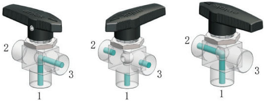
端口1和3连通 关断 端口1和2连通
